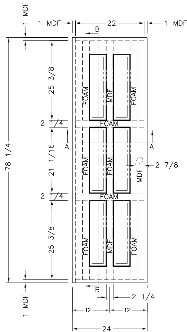
DOOR CONSTRUCTION
