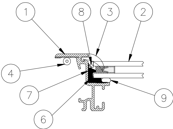
SECTION A-A SCALE : 4x
