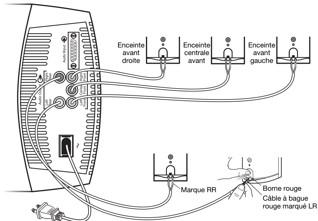
Module Acoustimass® 10
