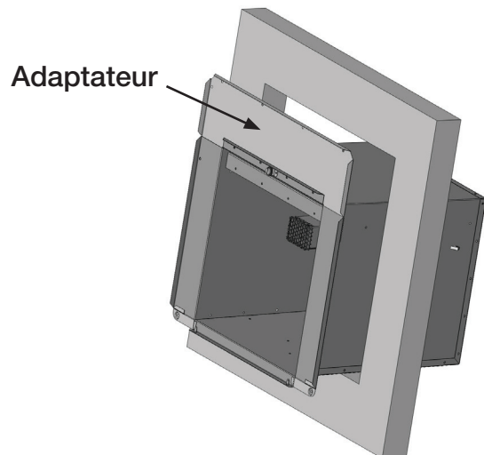
Installation dans l'ouverture d'un chauffe-eau de 10 gallons standard avec la trousse et l'adaptateur pour une grande porte.
