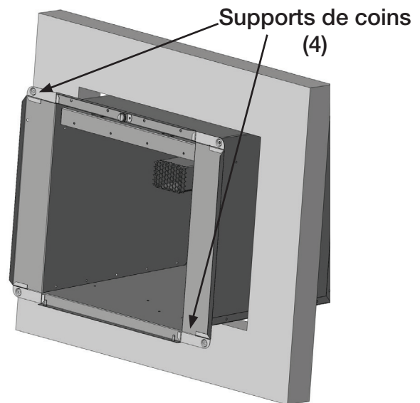
Installation dans l'ouverture d'un chauffe-eau de 6 gallons standard avec la trousse pour une porte standard
