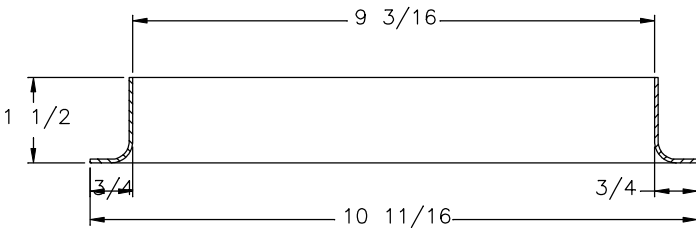
SECTION A-A (4X SCALE)
