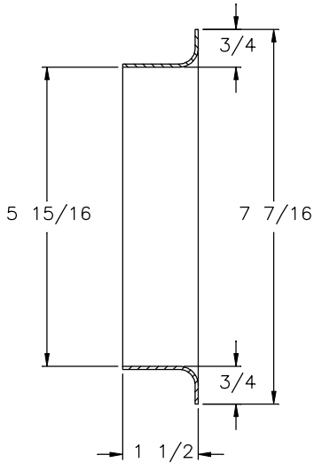
SECTION B-B (4X SCALE)
