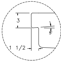
VIEW A SCALE: 2-1
