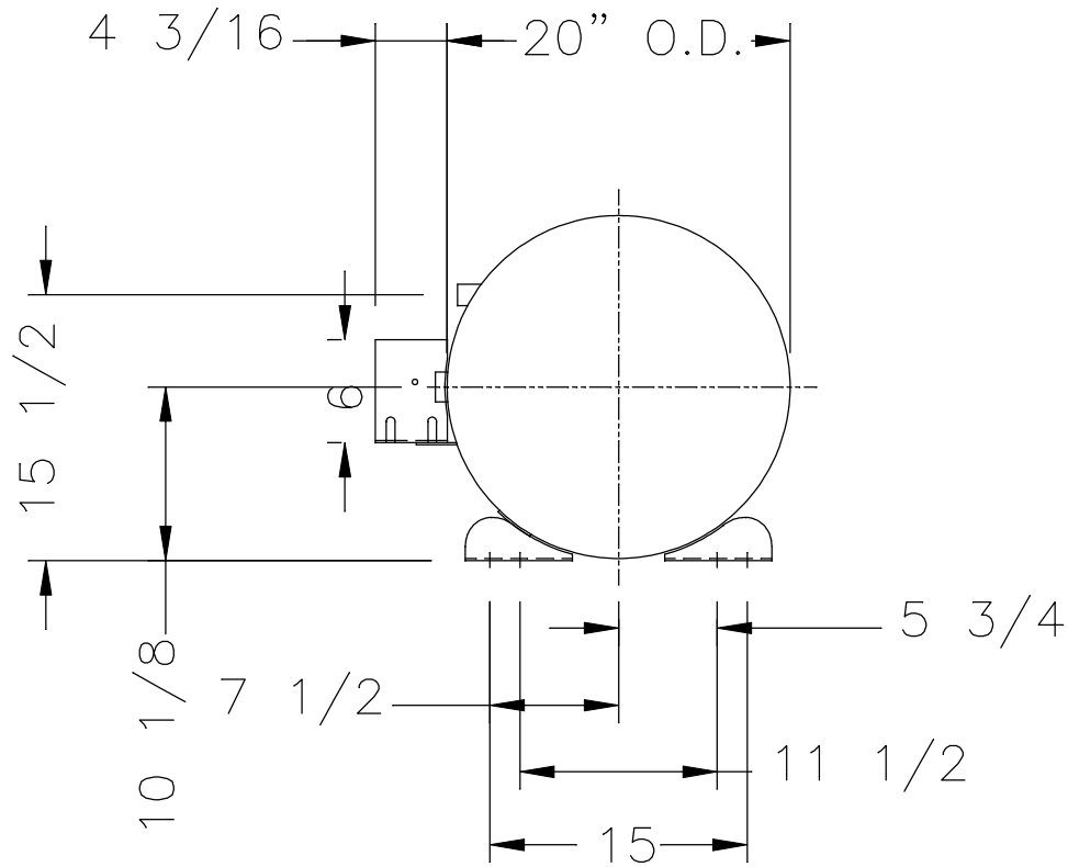
LP_TANK_SIDE
