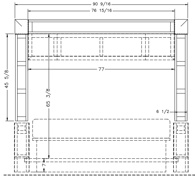
BEDROOM S-O FASCIA
