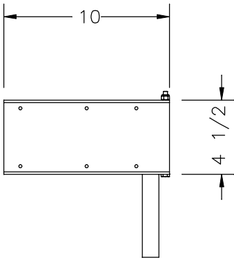
VIEW A-A
