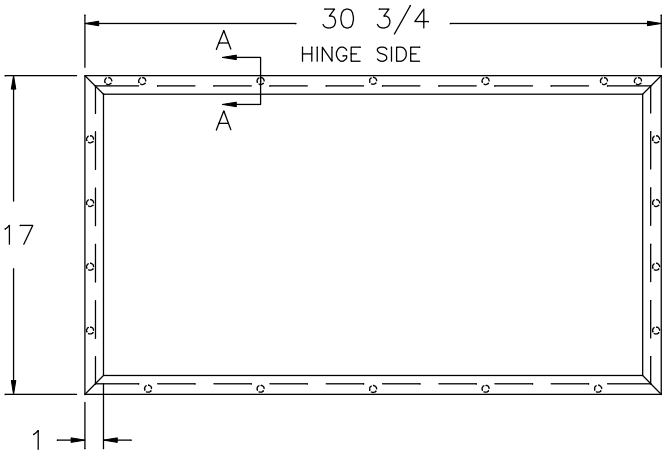
LOUVER FRAME
