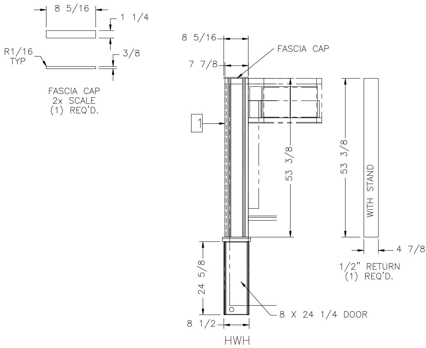
DS DINETTE ENTERTAINMENT S-O FASCIA
