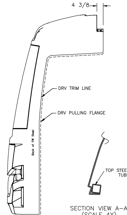
DOOR SIDE
