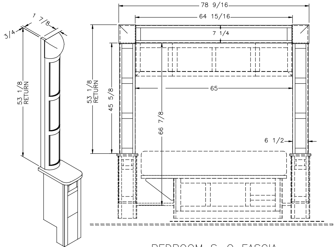
BEDROOM S-O FASCIA
