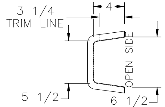
SIDE SECTION (D)
