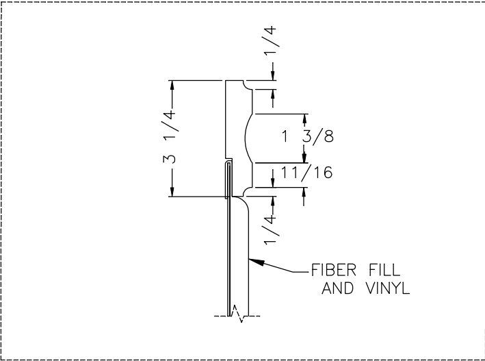
SECTION A—A SCALE: 4x
