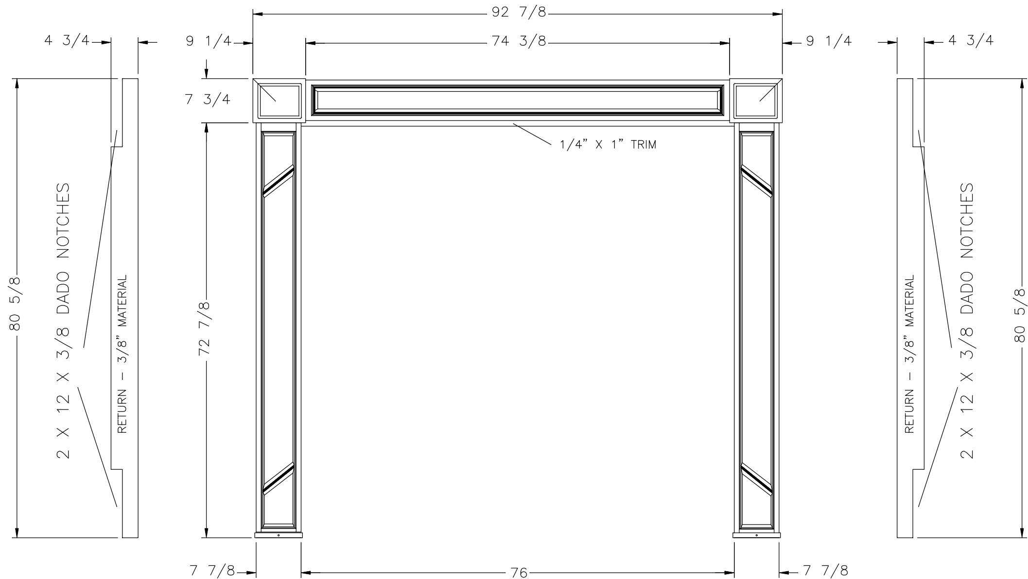
WARDROBE S-O FASCIA
