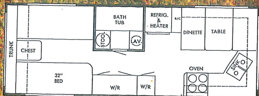
22' F.K. SIDE BATH
