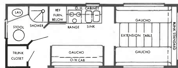
22 FT. TWIN GAUCHO
