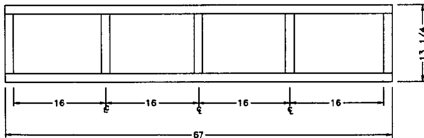
RISER 1
