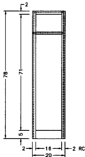
(1) 16 1/2 X 71 1/2 MIRROR DOOR
