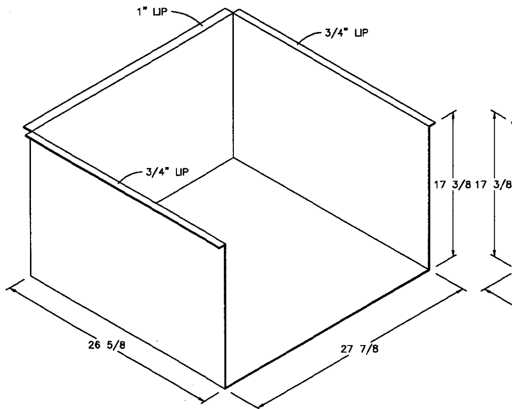
DOOR SIDE
