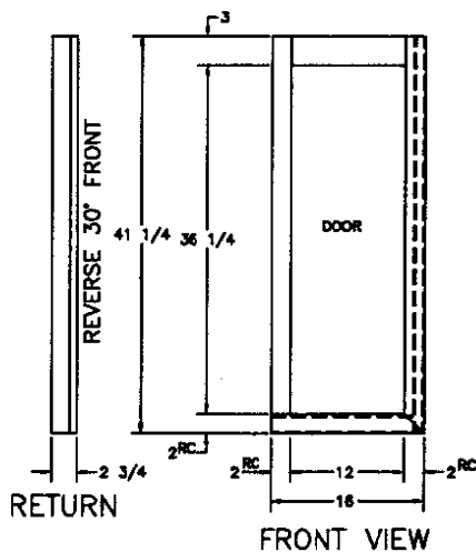
DOOR SIDE
