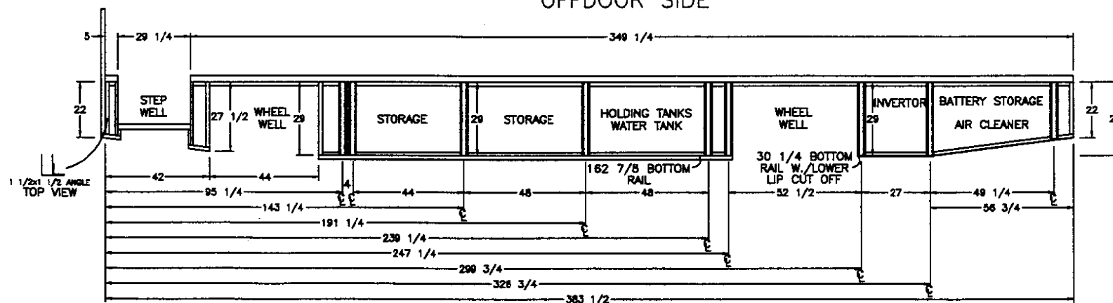
DOOR SIDE
