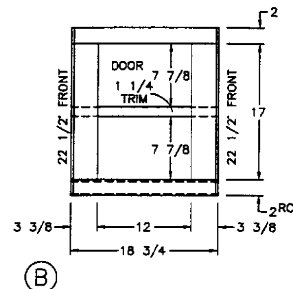
(1) 12 1/2x17 1/2 DOOR
