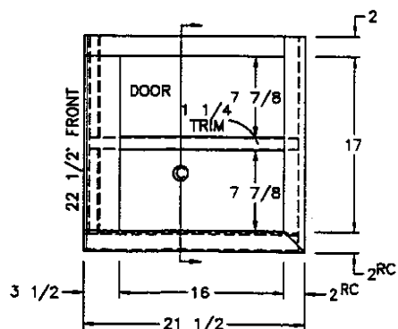
(1) 16 1/2x17 1/2 DOOR
