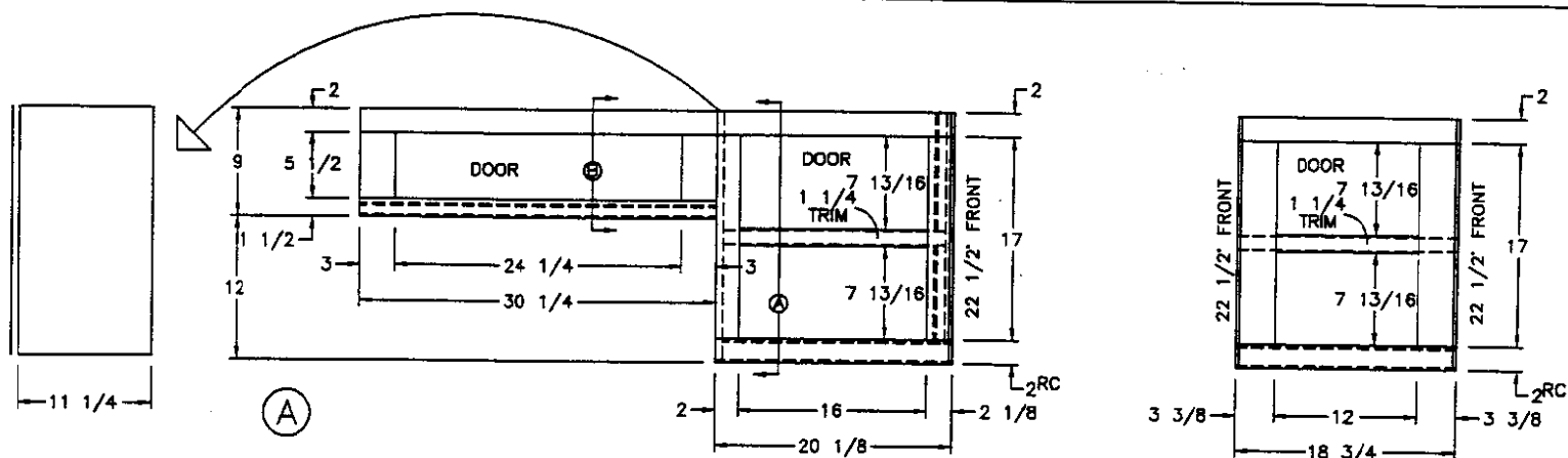
(1) 12 1/2x17 1/2 DOOR
