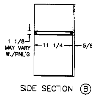
(1) 12 1/2x17 1/2 DOOR
