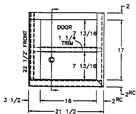
(1) 16 1/2x17 1/2 DOOR
