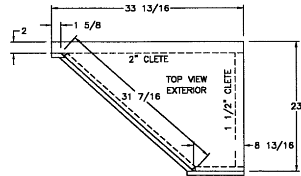
DOOR SIDE
