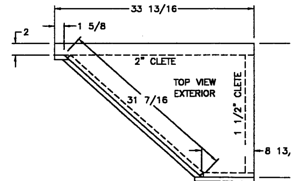
DOOR SIDE
