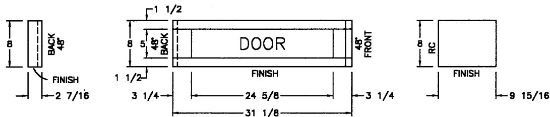
DOOR SIDE FRONTS (1) 25 1/8x5 1/2 DOOR
