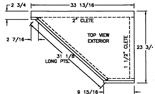
DOOR SIDE
