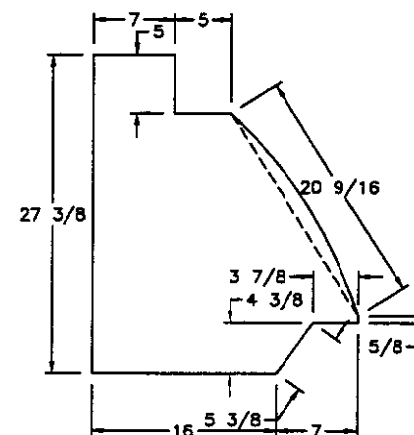
SIDE PER PATTERN
