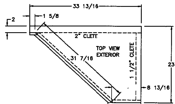
DOOR SIDE
