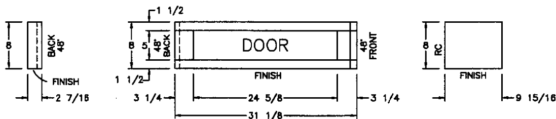
DOOR SIDE FRONTS (1) 25 1/8x5 1/2 DOOR
