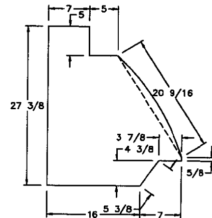
SIDE PER PATTERN
