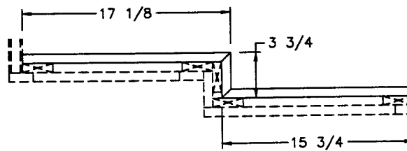
TOE-KICK
