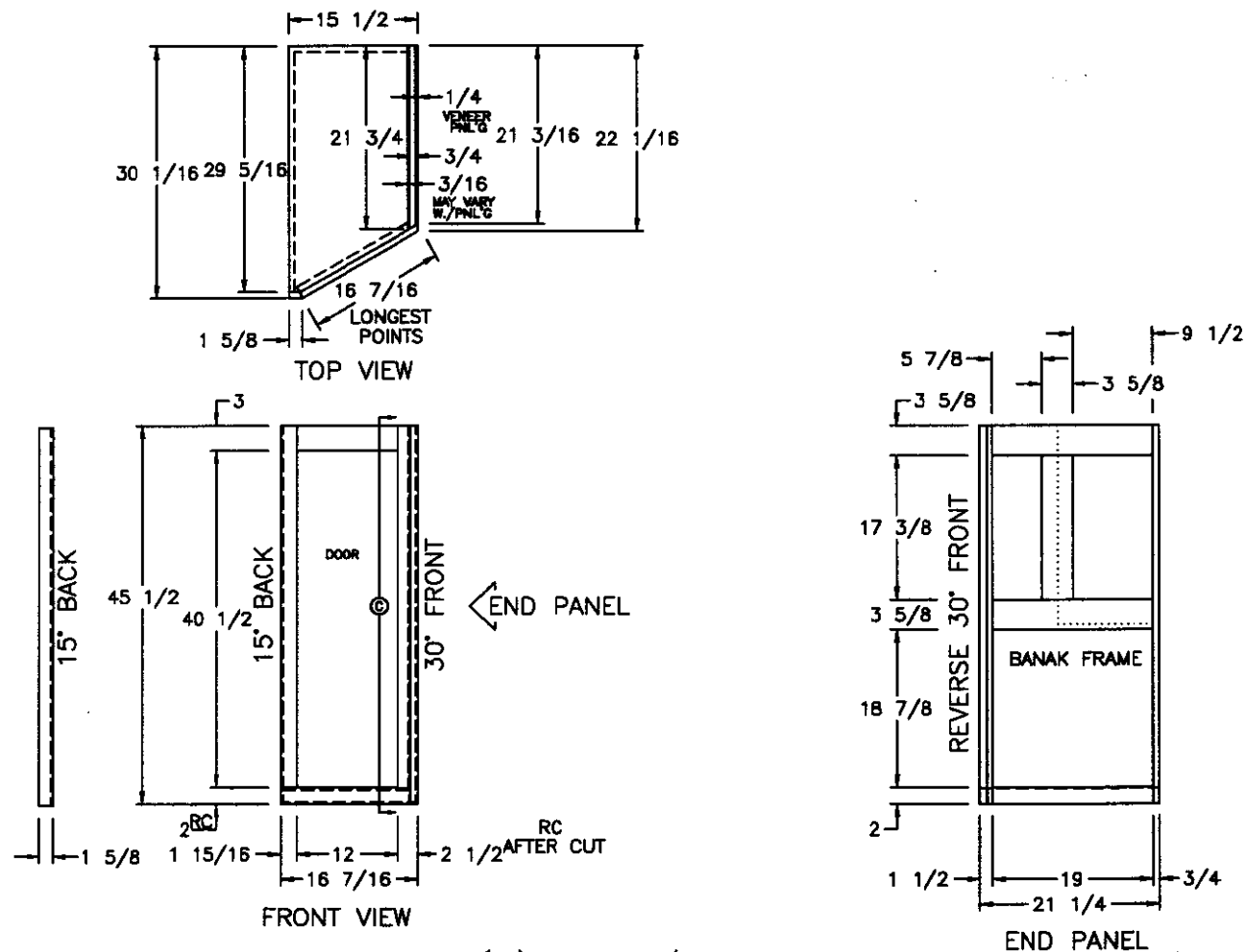
(1) 12 1/2x41 DOOR
