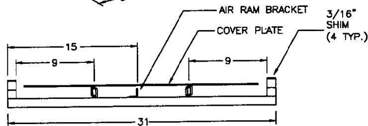
SEC. A-A
