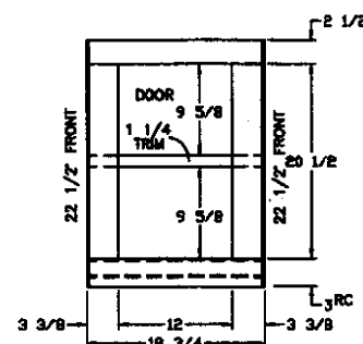
(1) 12 1/2x22 1/2 GLASS DOOR
