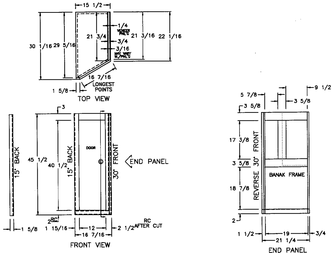
(1) 12 1/2x41 DOOR
