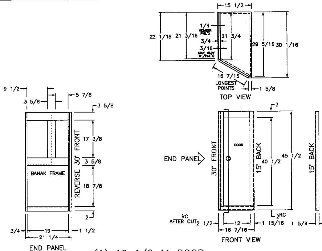
(1) 12 1/2x41 DOOR
