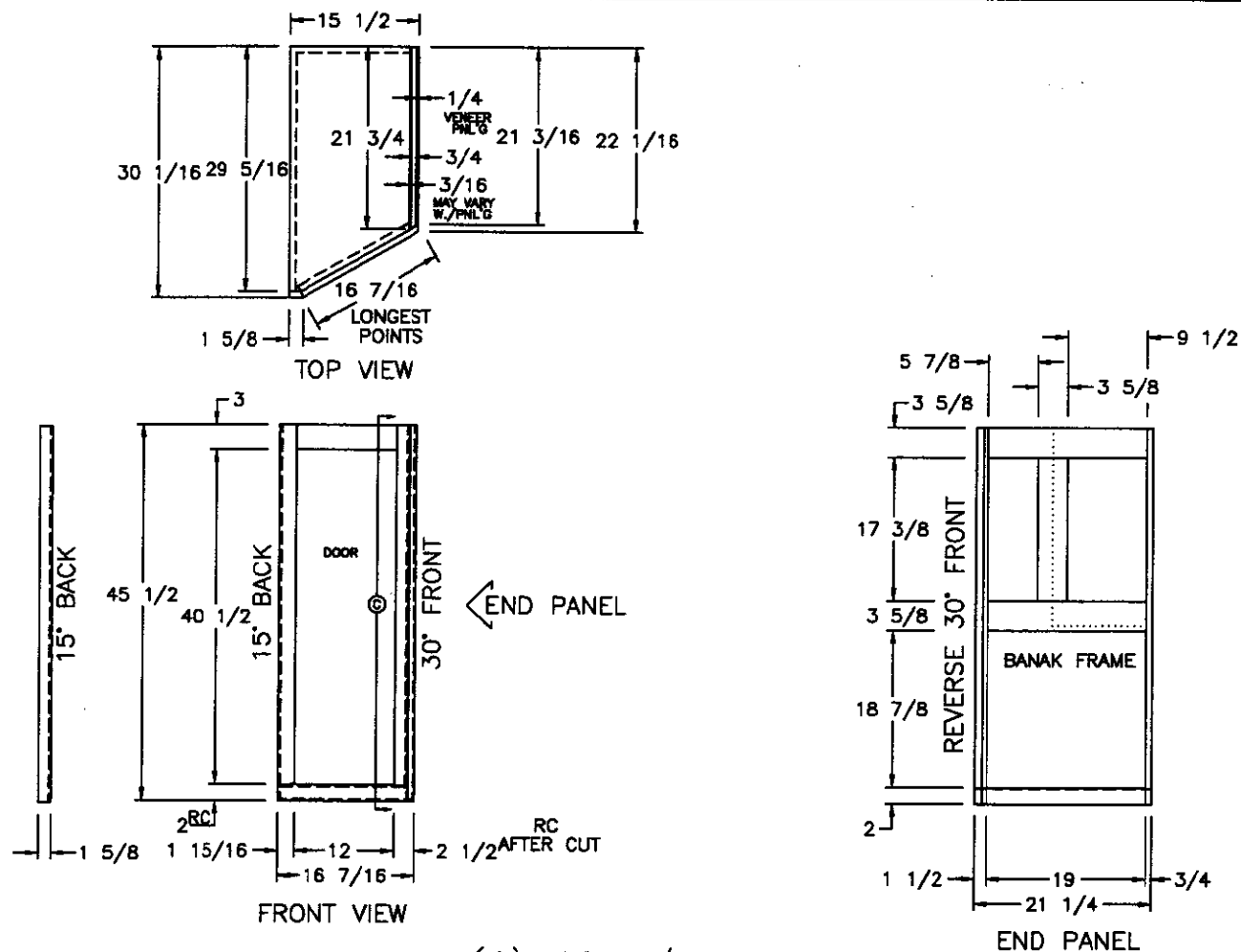
(1) 12 1/2x41 DOOR
