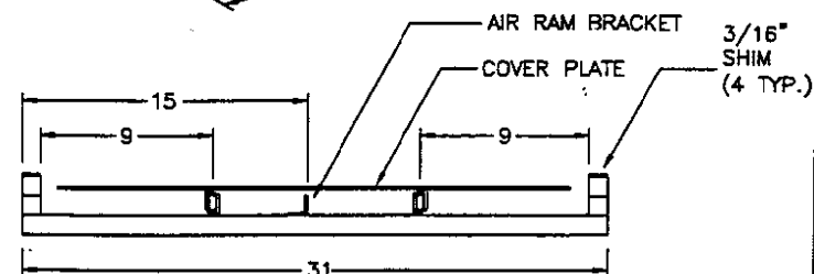
SEC. A-A
