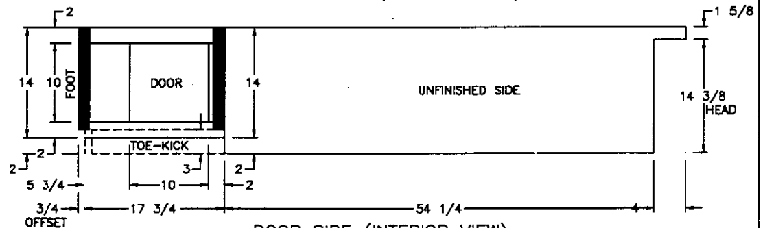
DOOR SIDE (INTERIOR VIEW)
