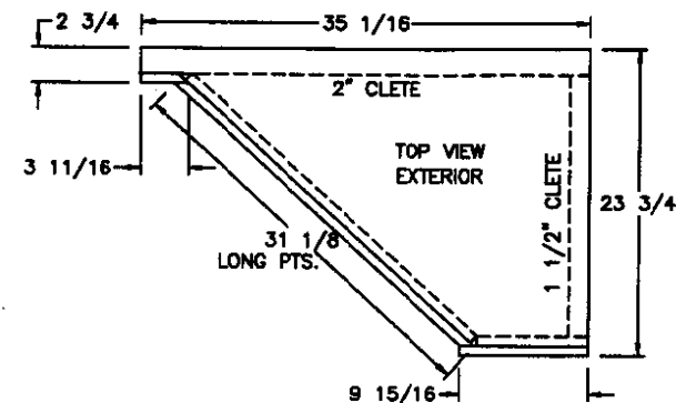
DOOR SIDE
