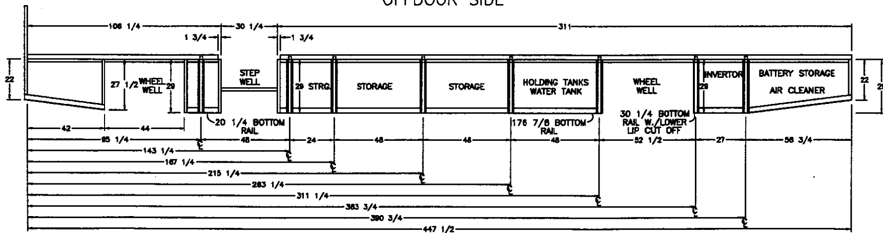
DOOR SIDE
