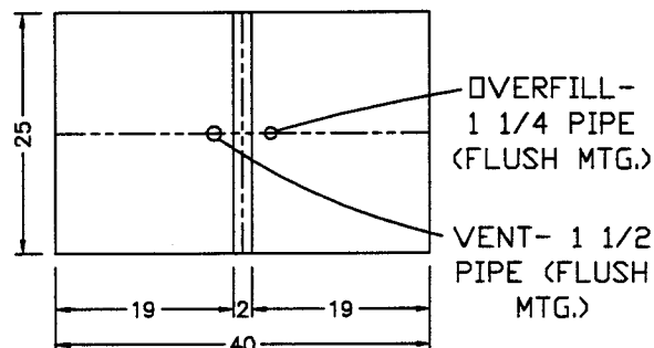
TOP
