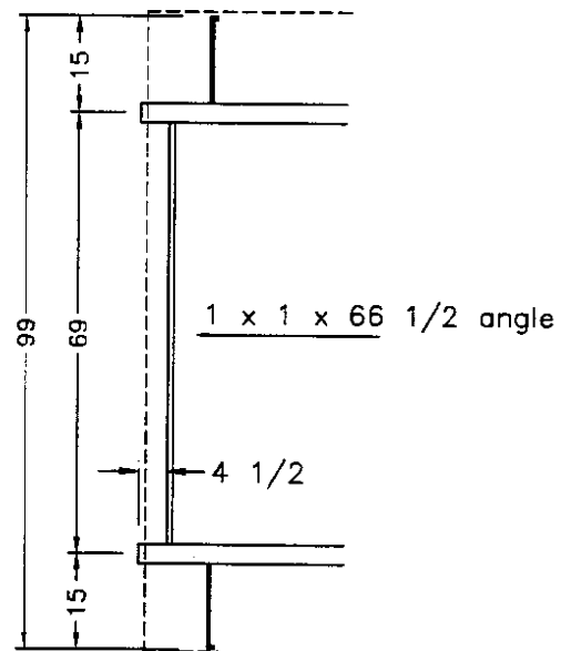
Aire 12" I-beam
