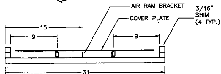
SEC. A-A
