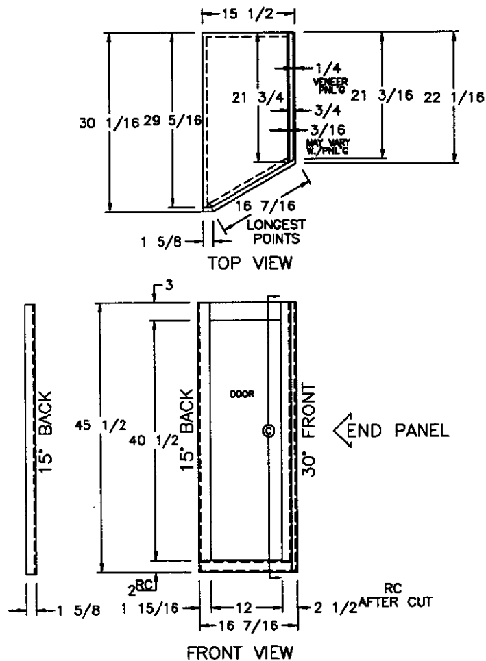
(1) 12 1/2x41 DOOR
