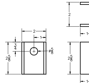
STOP ROD BRACKET ITEM-4 SCALE: 3X
