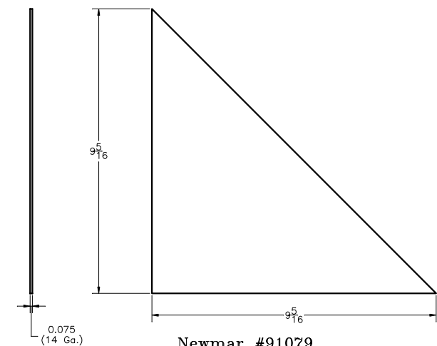
Newmar #91079 ITEM-1 3X Scale
