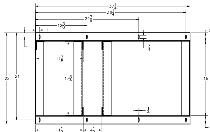
Newmar #91081 ITEM-3 3X Scale
