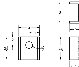
STOP ROD BRACKET ITEM-3 SCALE: 3X
