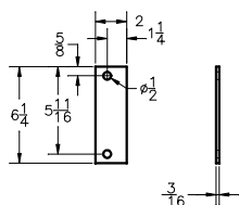
GUIDE PLATES ITEM-4 SCALE: 2X
