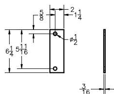
GUIDE PLATES ITEM-5 SCALE: 2X
