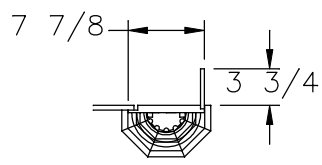
NON-FLUSH HWH COLUMN
