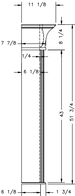
VERT COLUMN SIDE VIEW DOOR SIDE TOP OF END TABLE
