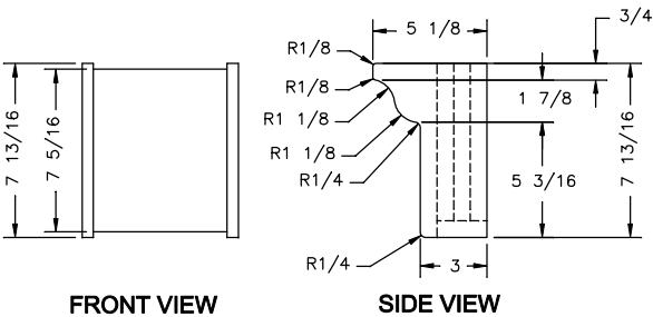
POCKET DOOR MA 4102 JAMB CONFIGURATION
