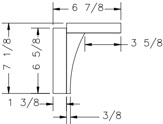
SECTION D-D SCALE: 2x
