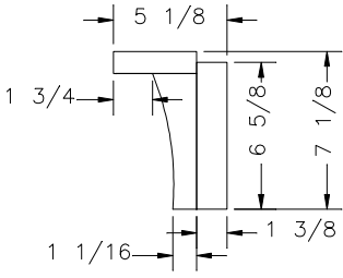
SECTION G-G SCALE: 2x
