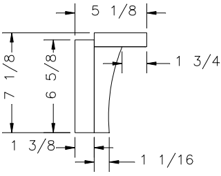
SECTION F-F SCALE: 2x
