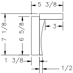
SECTION E-E SCALE: 2x
