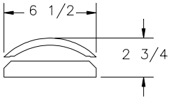
SECTION C-C SCALE: 2x
