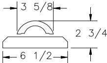
SECTION B-B SCALE: 2x
