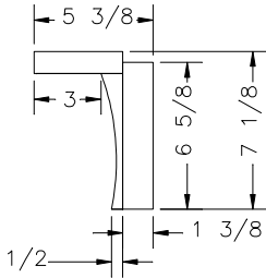
SECTION H-H SCALE: 2x
