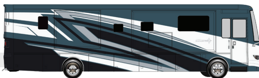
ALTAIR
