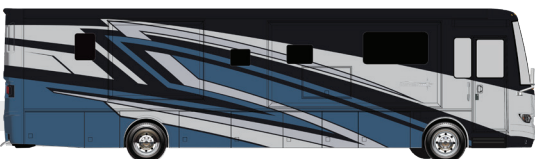
DENEb
