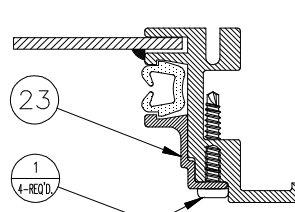
SECTION D-D SCALE: FULL
