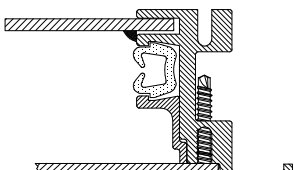
SECTION C-C SCALE: FULL
