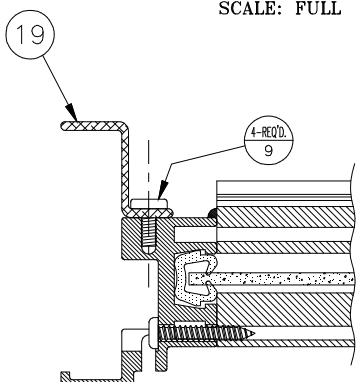
SECTION B-B SCALE: FULL
