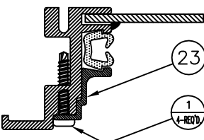
SECTION D-D SCALE: FULL
