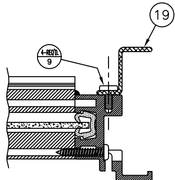
SECTION B-B SCALE: FULL
