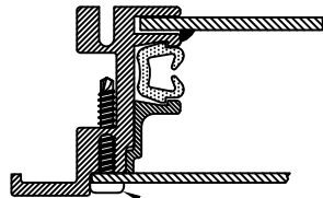
SECTION C-C SCALE: FULL
