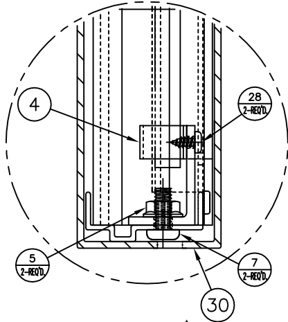
DETAIL E SCALE: FULL
