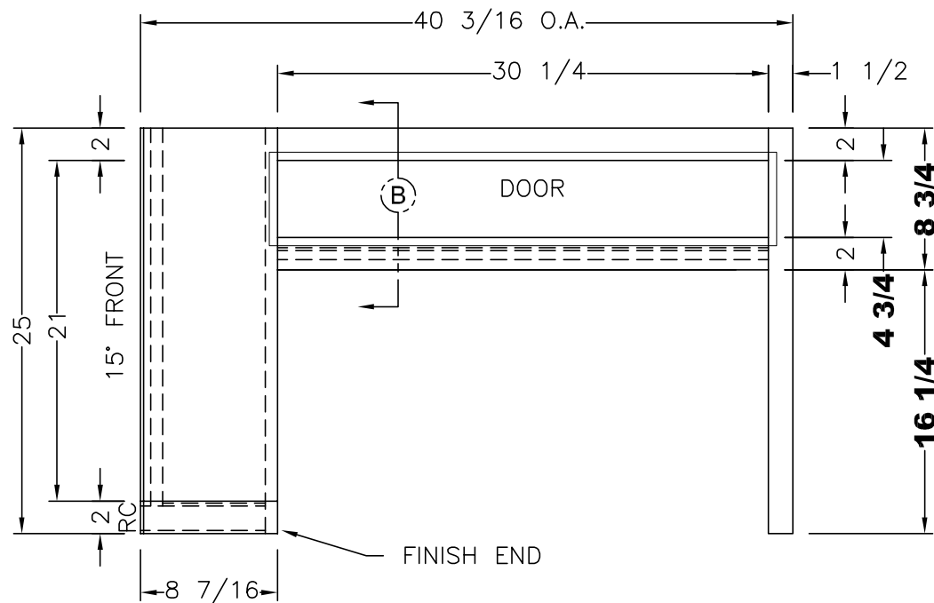
VIEW (D)
