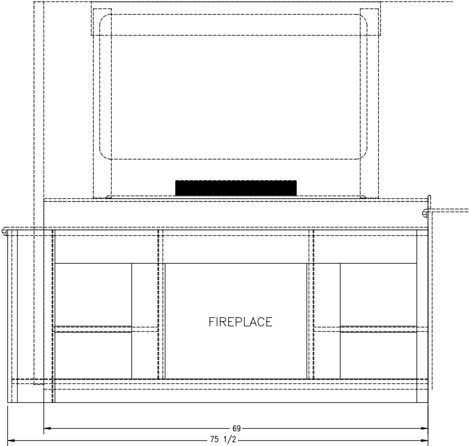
ELEVATION
