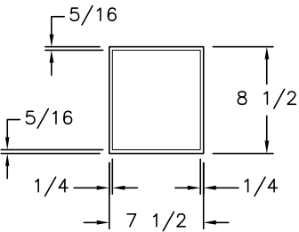
DOOR OVERLAY
