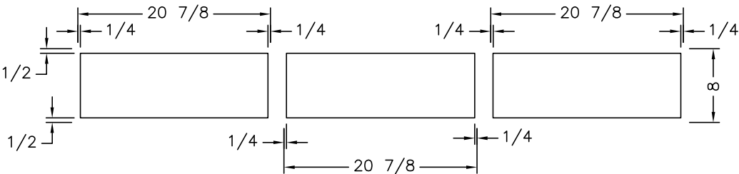
DOOR OVERHANGS
