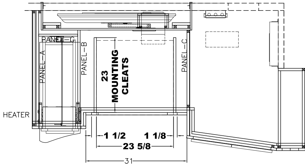
PLAN (J520)(J525)
