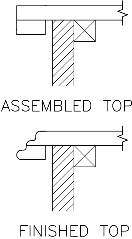
EDGE DETAIL
