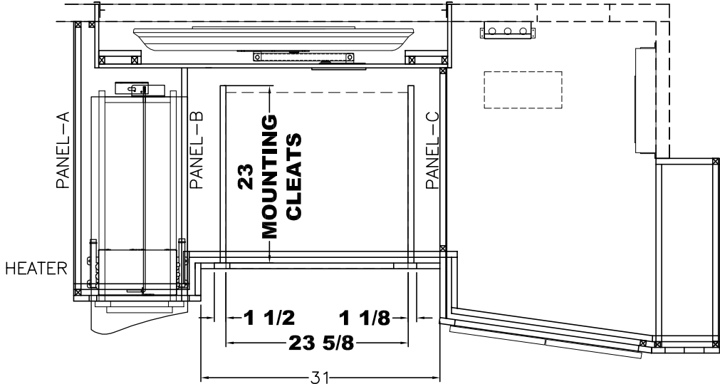
ⓑ PLAN (J525)
