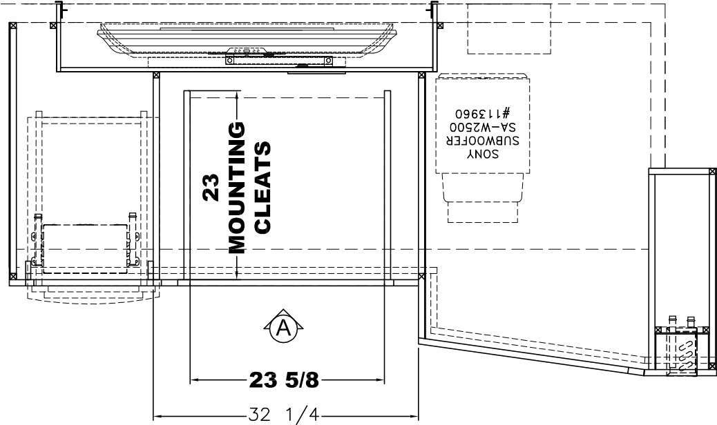
PLAN (J525)
